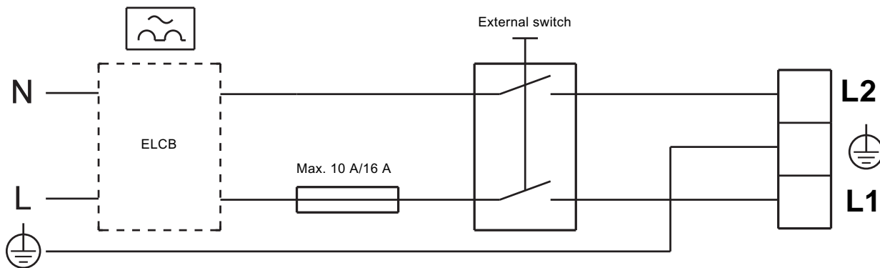
Fig. 17 1 x 230 V +/-10 %, 50/60 Hz
